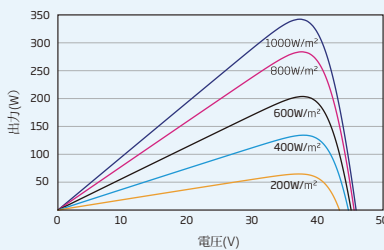
PVモジュール (345W) のP-V 曲線
