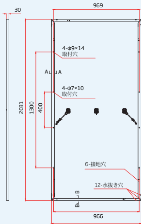
背面図
